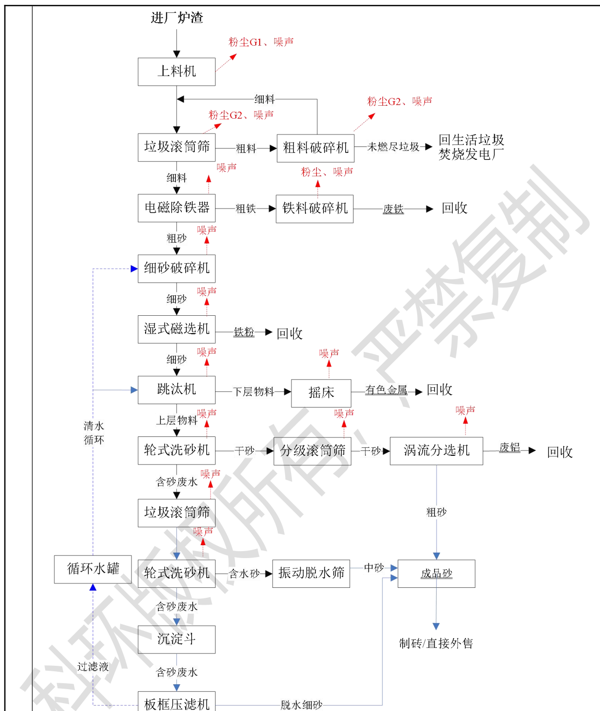
图 1 炉渣处理与资源化利用生产线生产工艺流程及产污环节图
