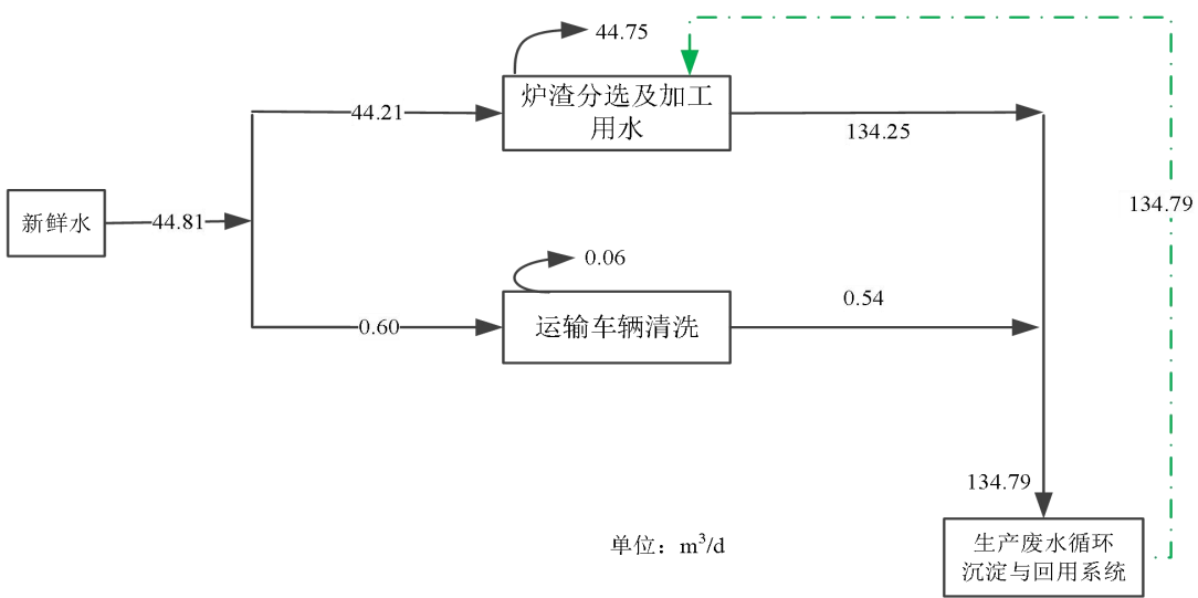
图 3 本项目水平衡图
