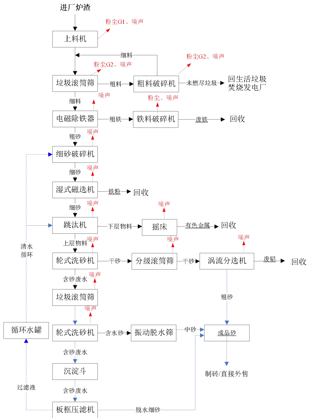
图 1 炉渣处理与资源化利用生产线生产工艺流程及产污环节图
