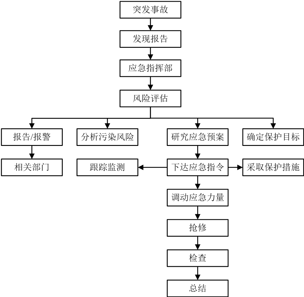
图 8 应急响应程序框图
