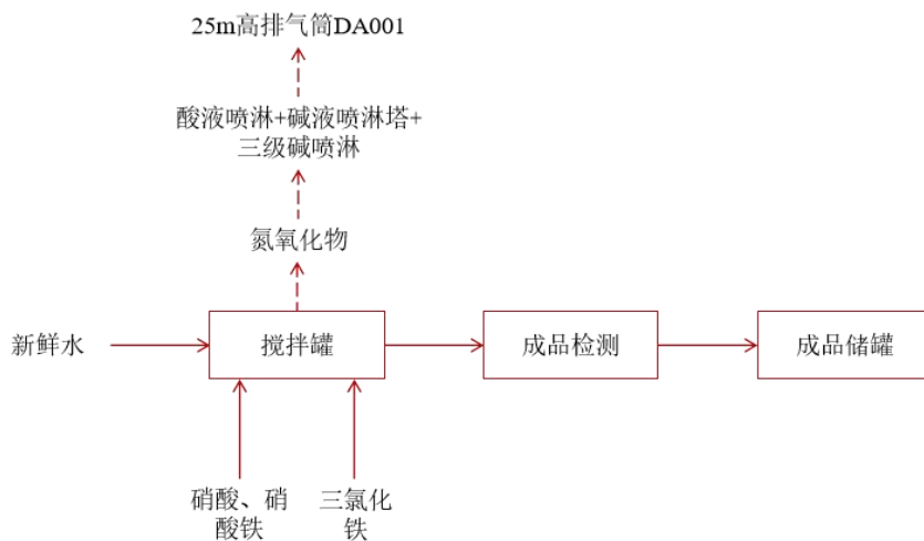
图 4 退锡水生产工艺流程及产污环节
