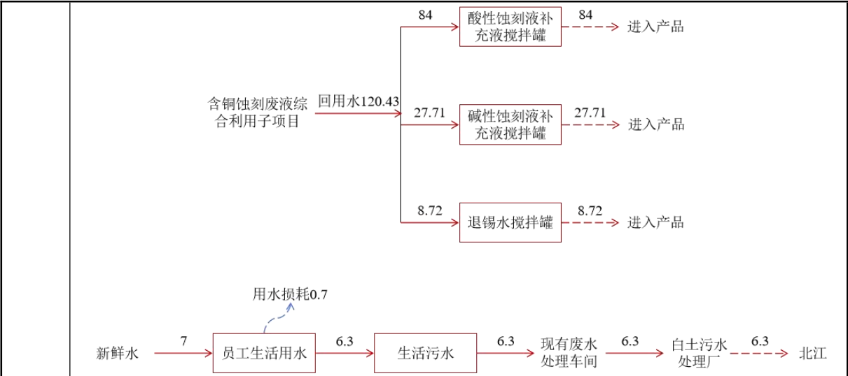
图 1 扩建项目用水平衡图
