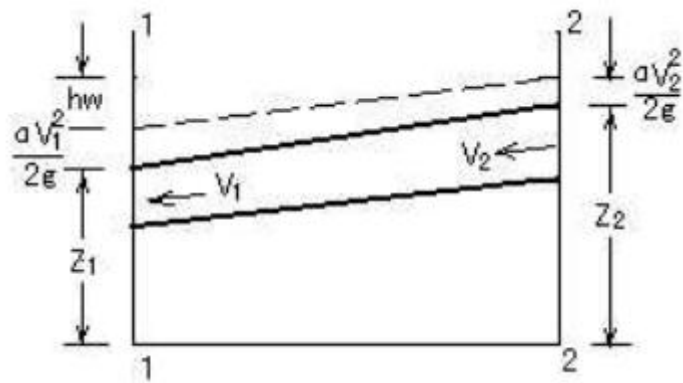
图 5.3-2 计算简图
