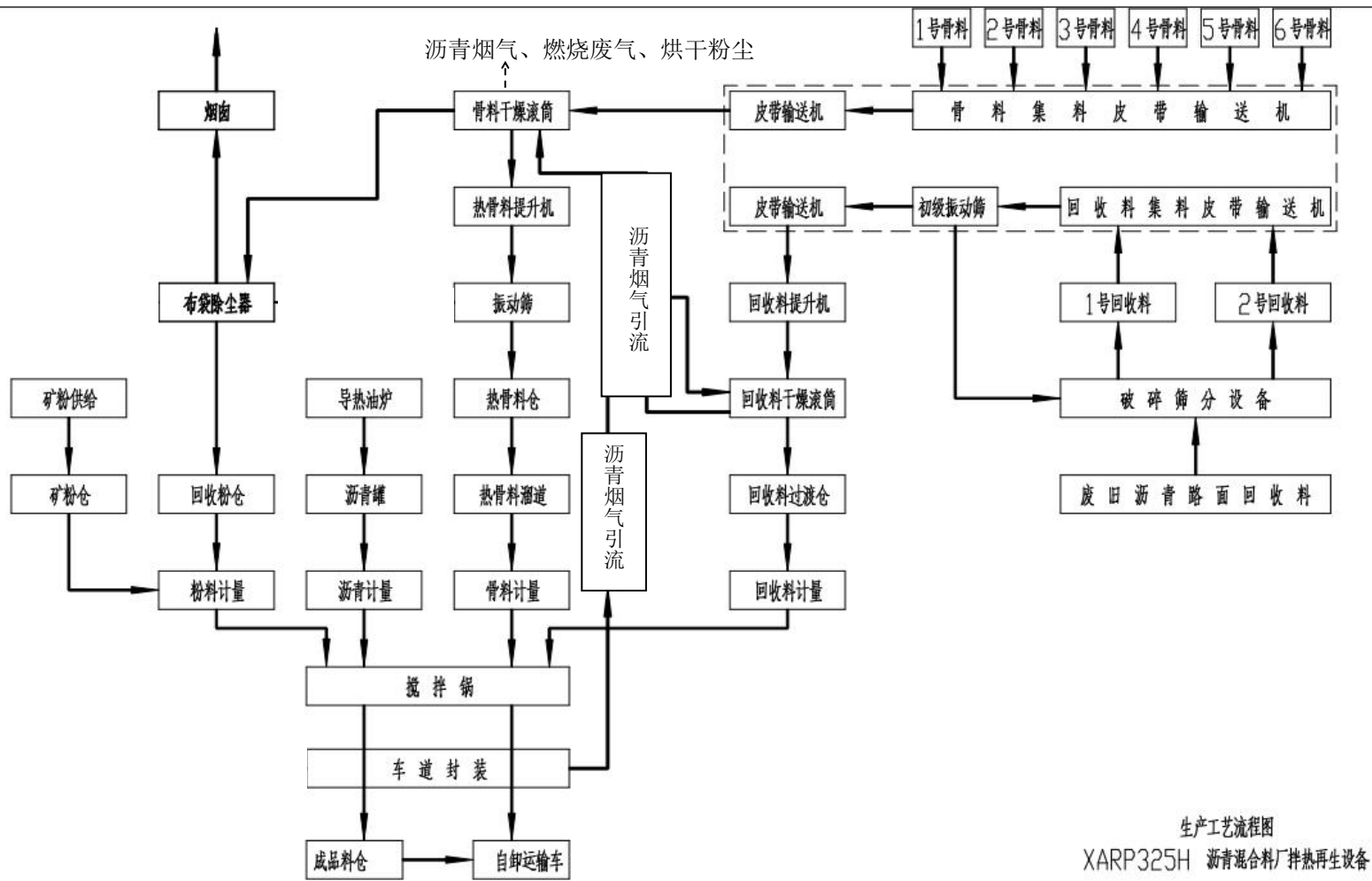
图 2-2 本项目营运期工艺流程图
