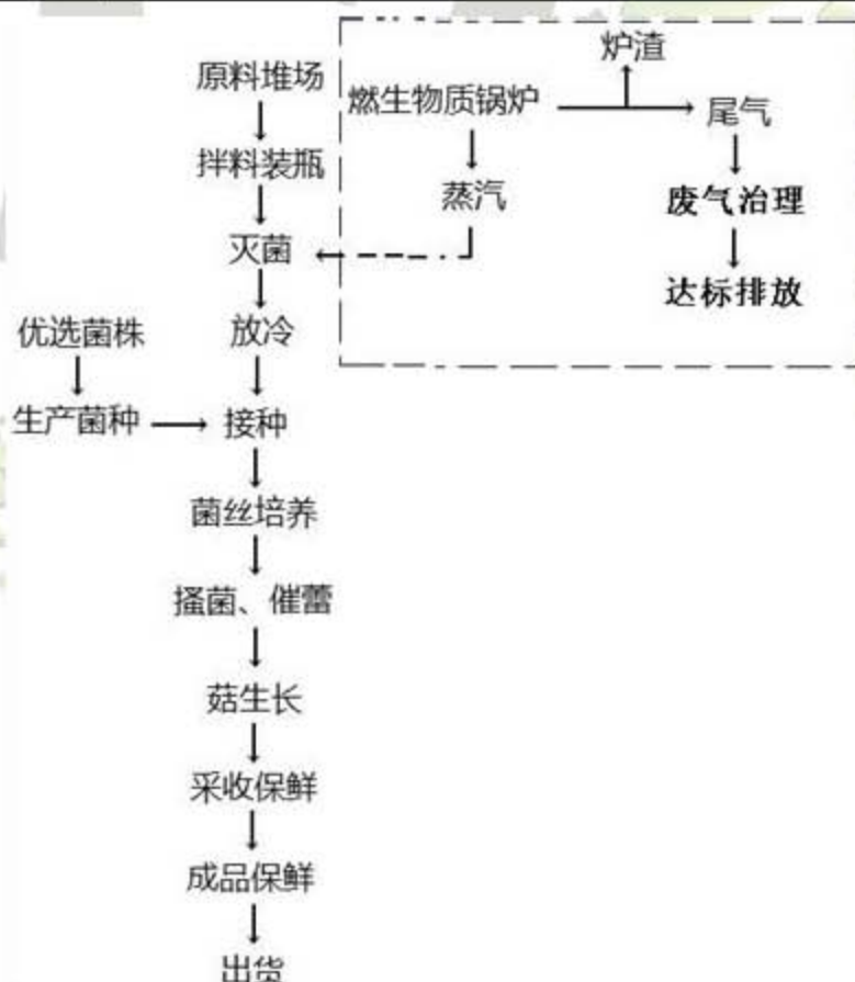
图 2-6 韶关市星河生物科技有限公司生产工艺流程图
