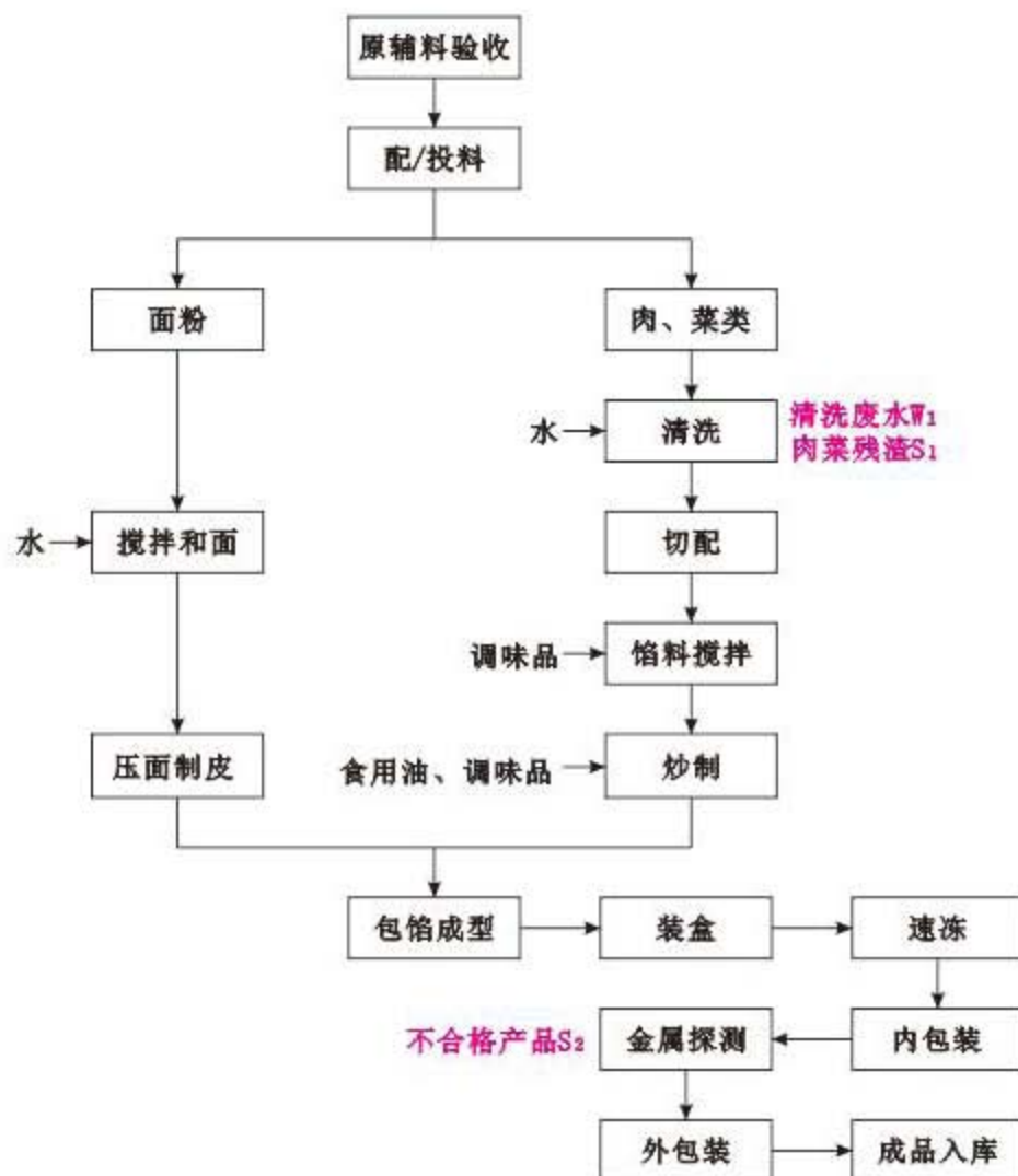
图 2-3 速冻饺子生产工艺流程及产污环节图
