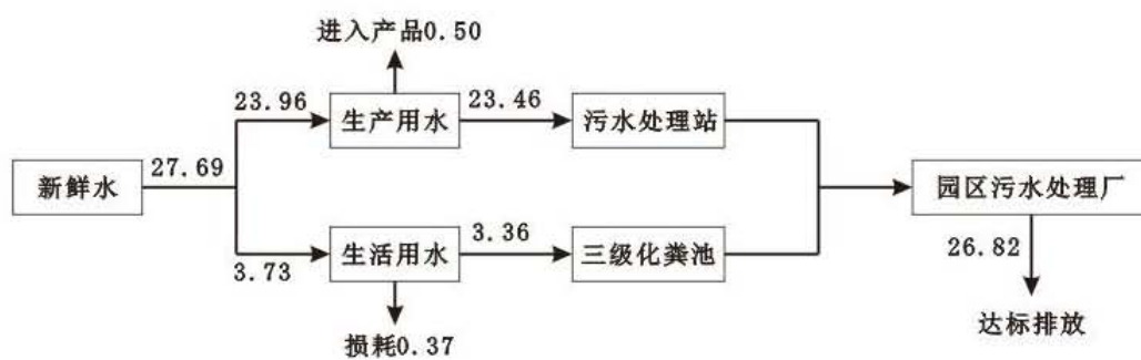
图 2-1 项目用水平衡图（单位：m³/d）
