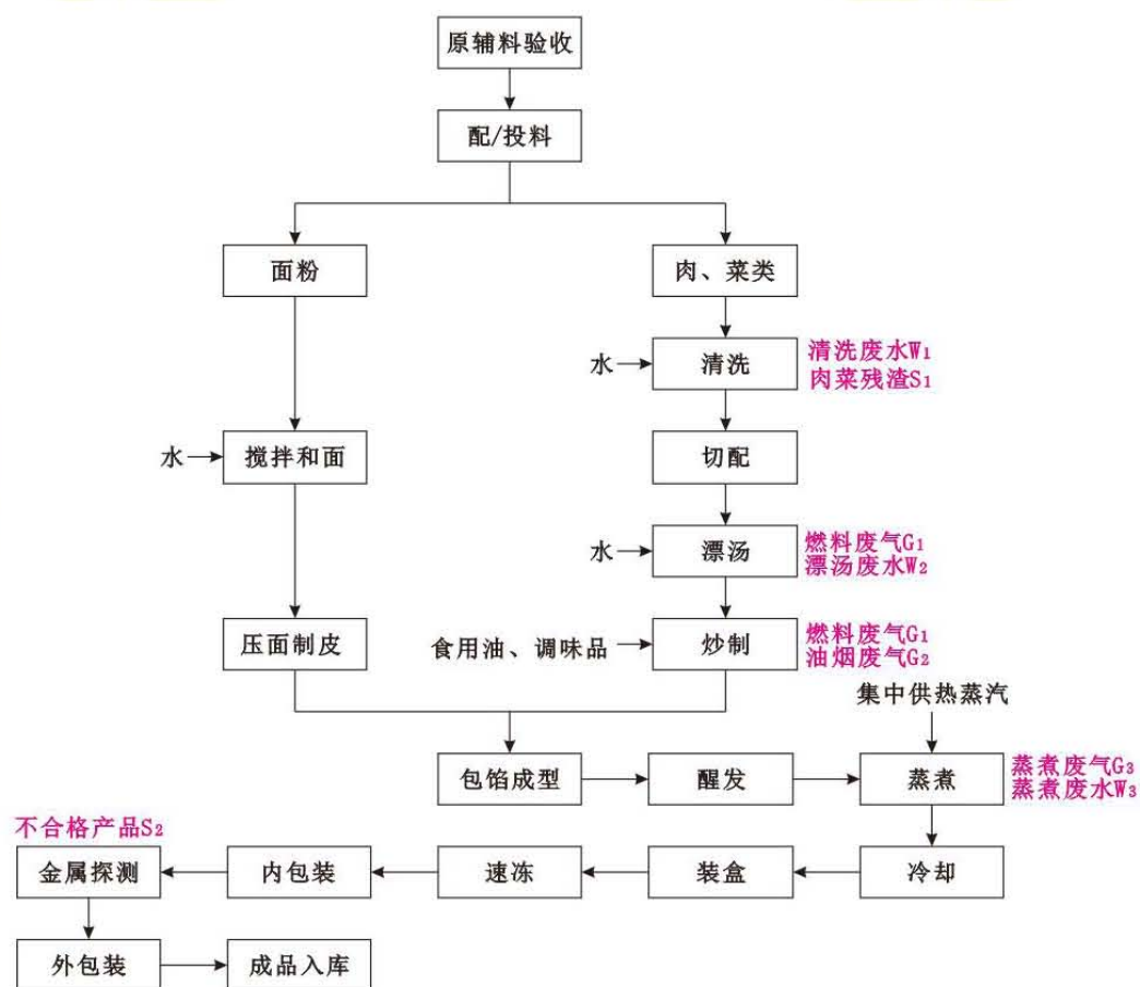
图 2-2 速冻包子生产工艺流程及产污环节图
