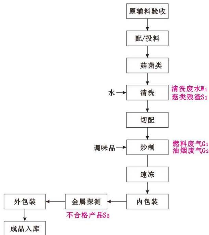
图 2-5 菇菌类预制菜生产工艺流程及产污环节图
