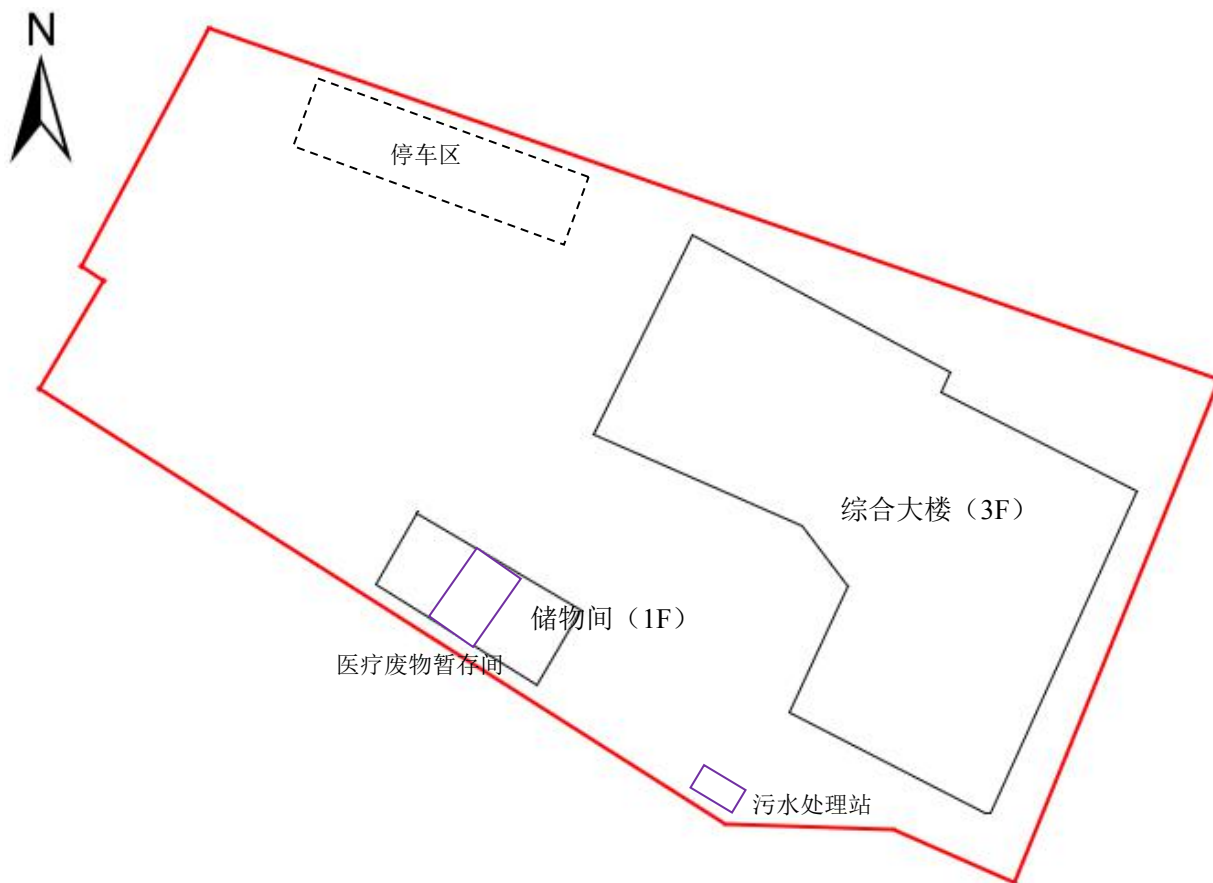
图 1-2 项目平面布置图
