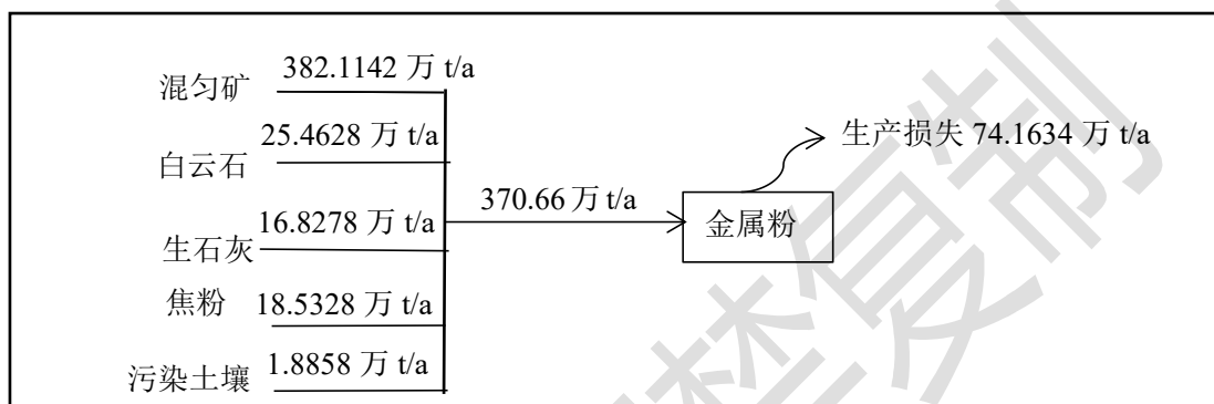
图 2-2 5 号烧结机技改后物料平衡图
