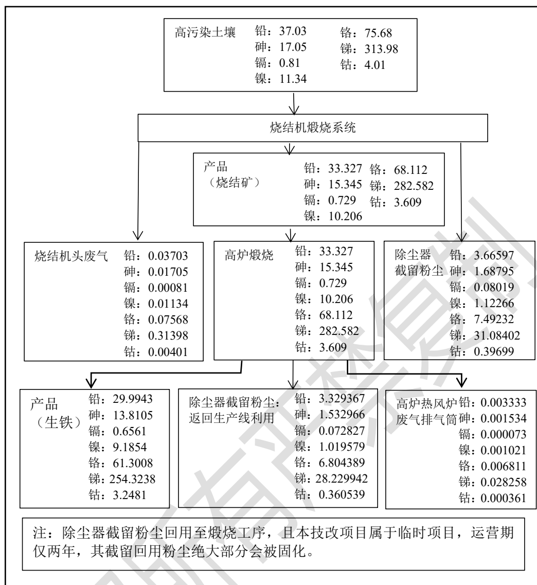
图 2.3-1 技改项目新增重金属平衡图 (t/a)
