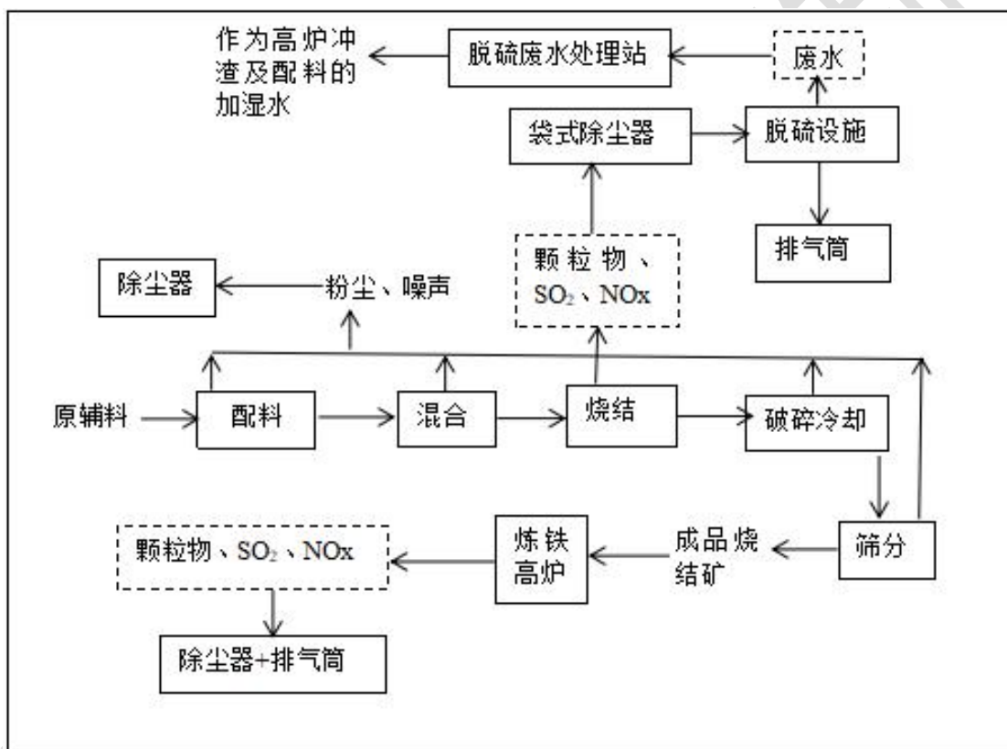
图 2-5 现有项目工艺流程图及产排污环节
