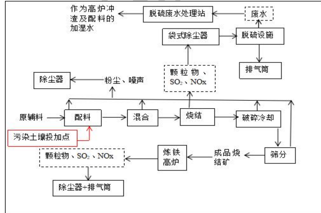
图 2.2-1 技改项目生产工艺及产污节点图
