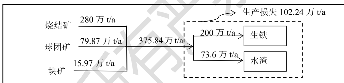
图 2-3 7 号高炉技改前后物料平衡图（技改前后未发生变化）
