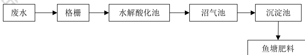
图 3-5 废水处理工艺流程图
