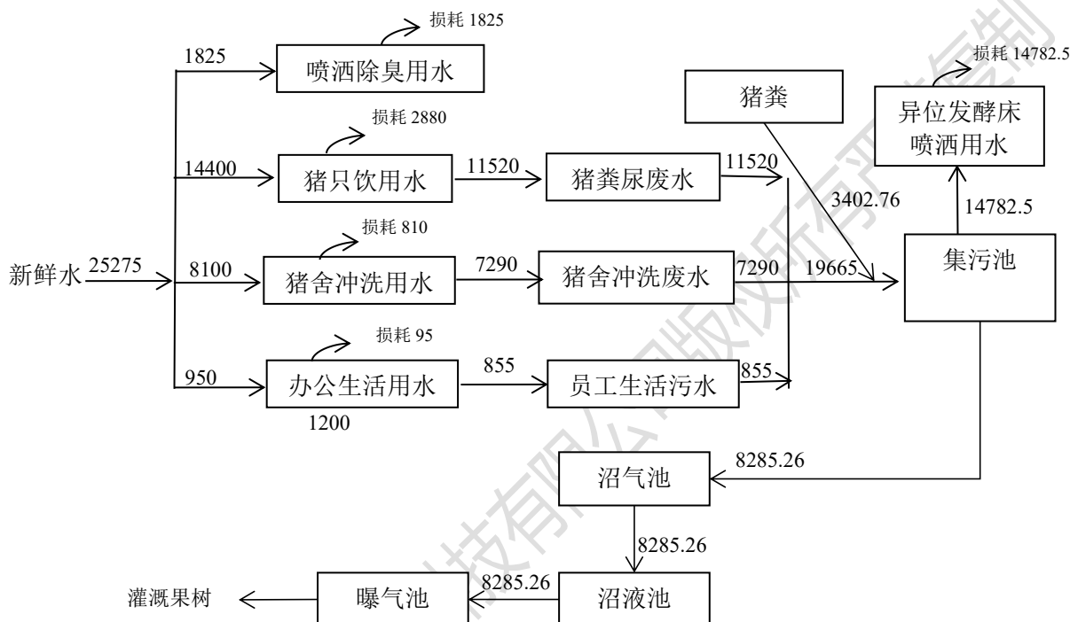
图 4-7 水平衡图 (单位: m 3 /a)
