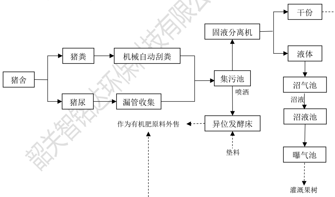
图 4-4 清粪及粪污处理工艺流程图
