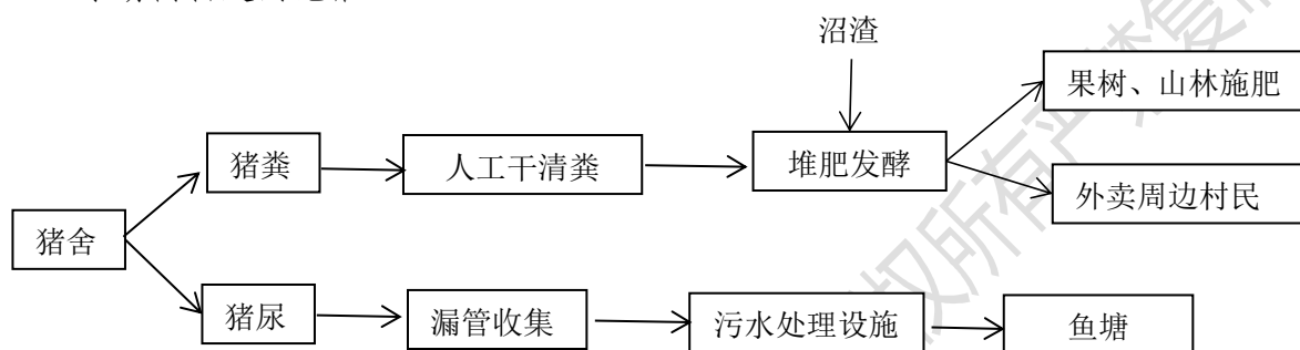
图 3-4 清粪及粪污处理工艺流程图
