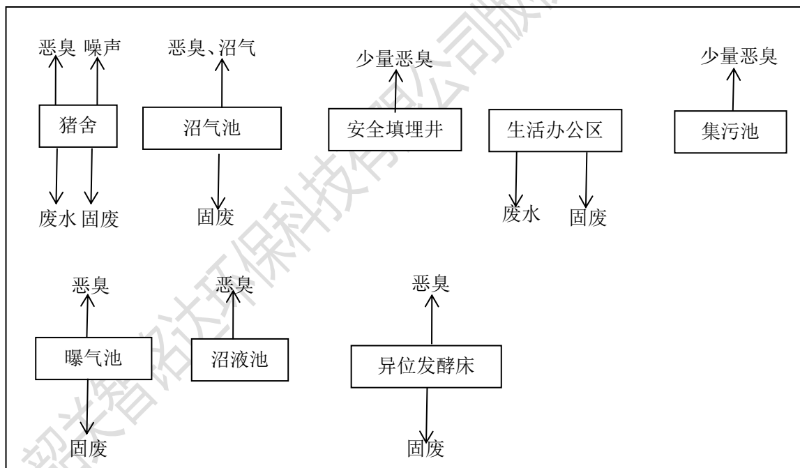
图 4-6 项目产污节点图
