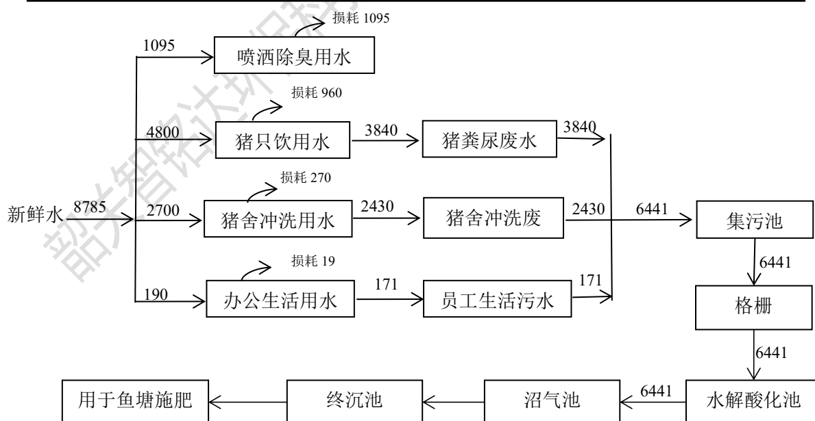
图 3-6 水平衡图 (单位: m 3 /a)
