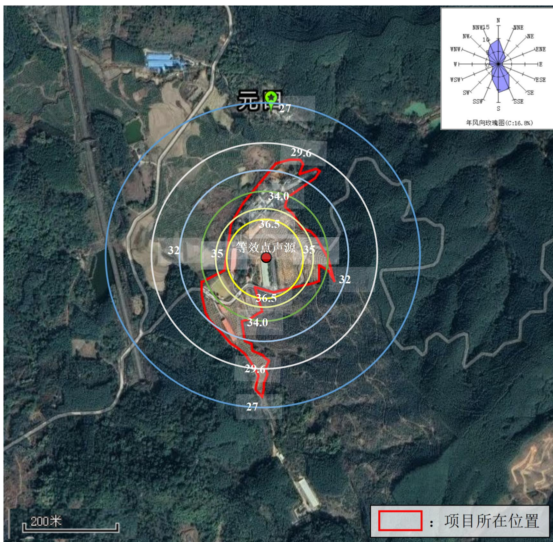
图 7-5 项目夜间噪声贡献值等值线图（单位：dB（A））
