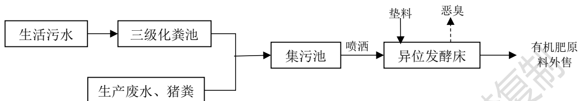
图 4-5 “异位发酵床”处理流程及产污环节图
