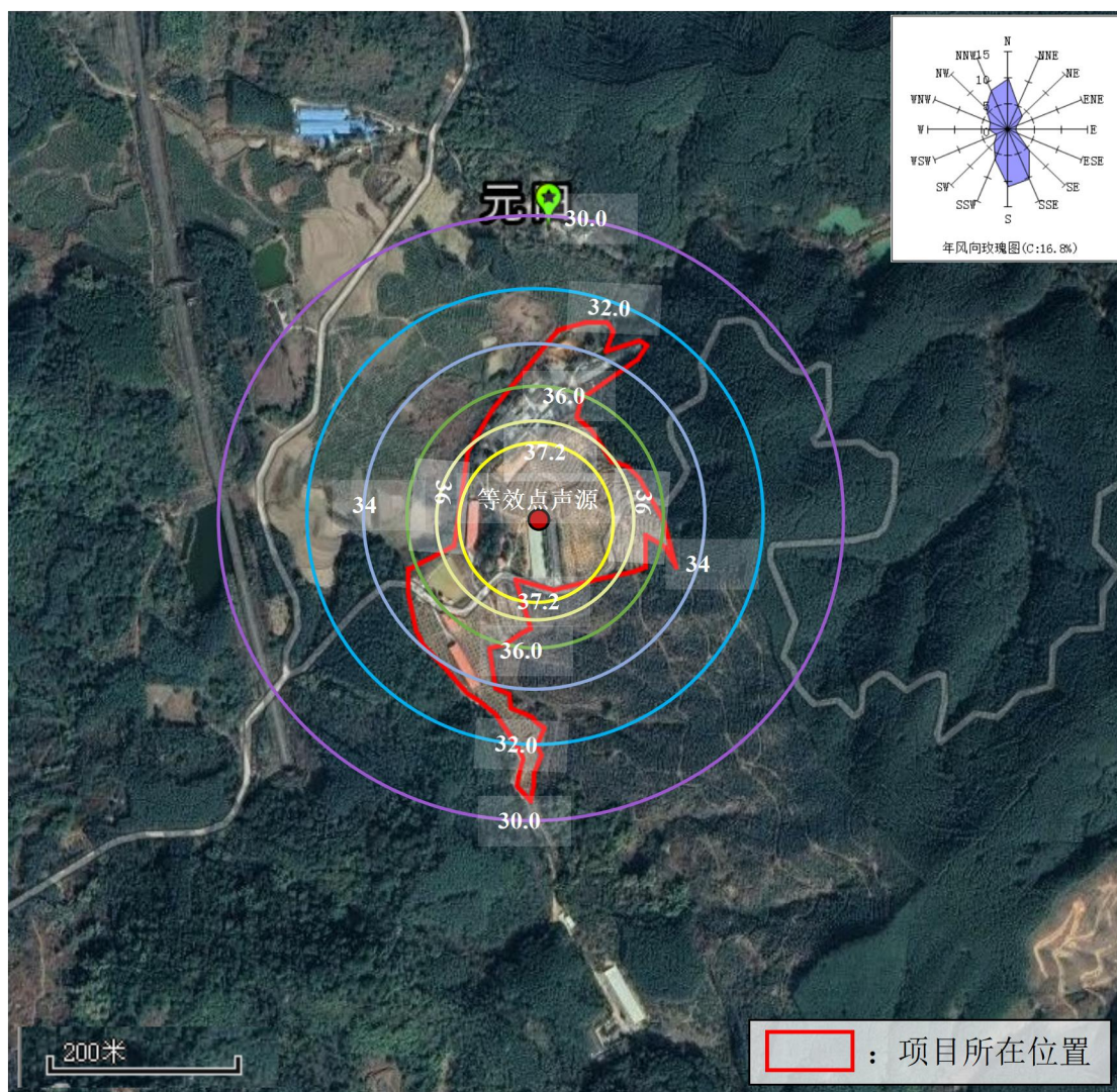
图 7-4 项目昼间噪声贡献值等值线示意图（单位：dB（A））
