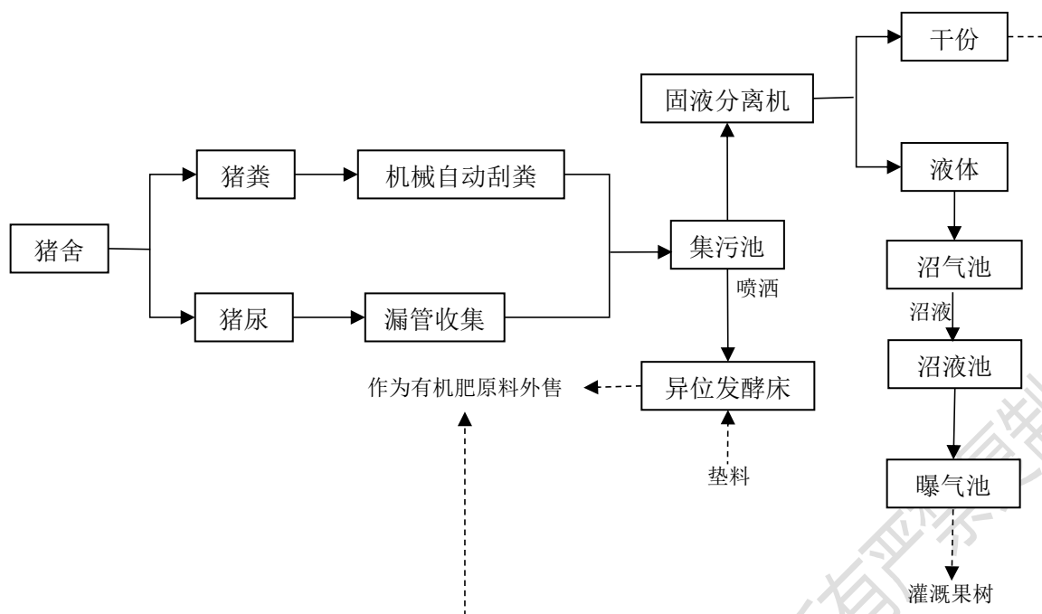
图 4-8 废水处理工艺流程图
