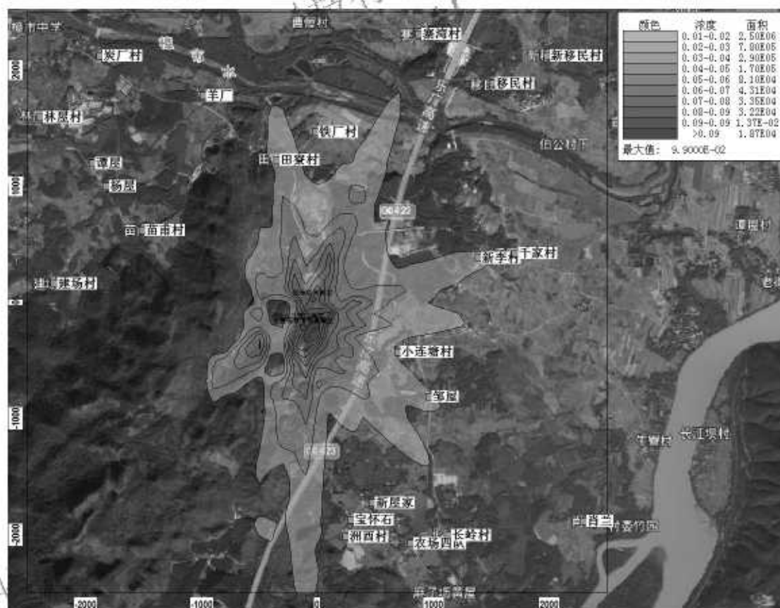
图 5-6 非正常排放情况下新增污染源 \text{NH}_3 小时平均浓度最大值分布图
