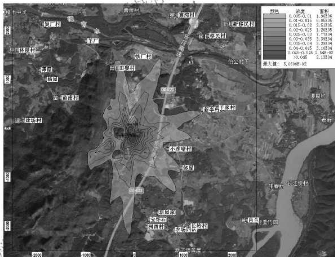
图 5-2 正常排放情况下新增污染源 NH 3 小时平均浓度最大值分布图
