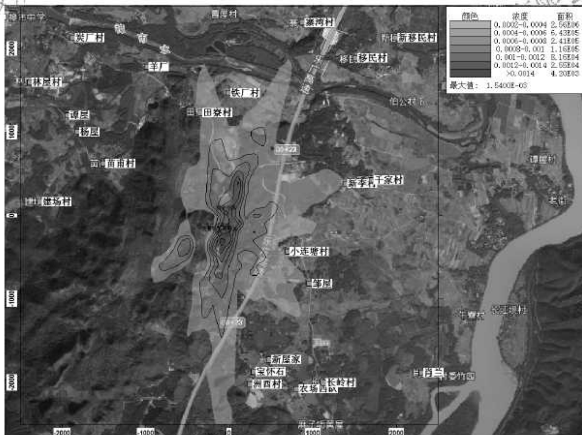
图 5-3 正常排放情况下新增污染源 H 2 S 小时平均浓度最大值分布图
