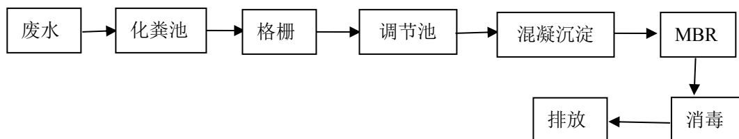
图 7-1 本项目废水处理工艺流程图
