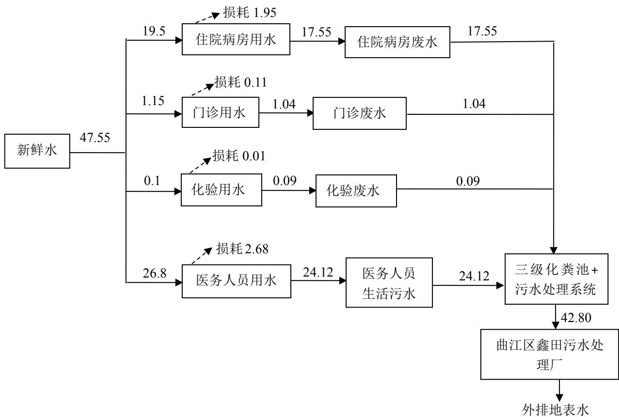
图 5-1 项目水平衡图 单位：m³/d
